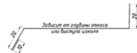
Рис. 1. Отлив
